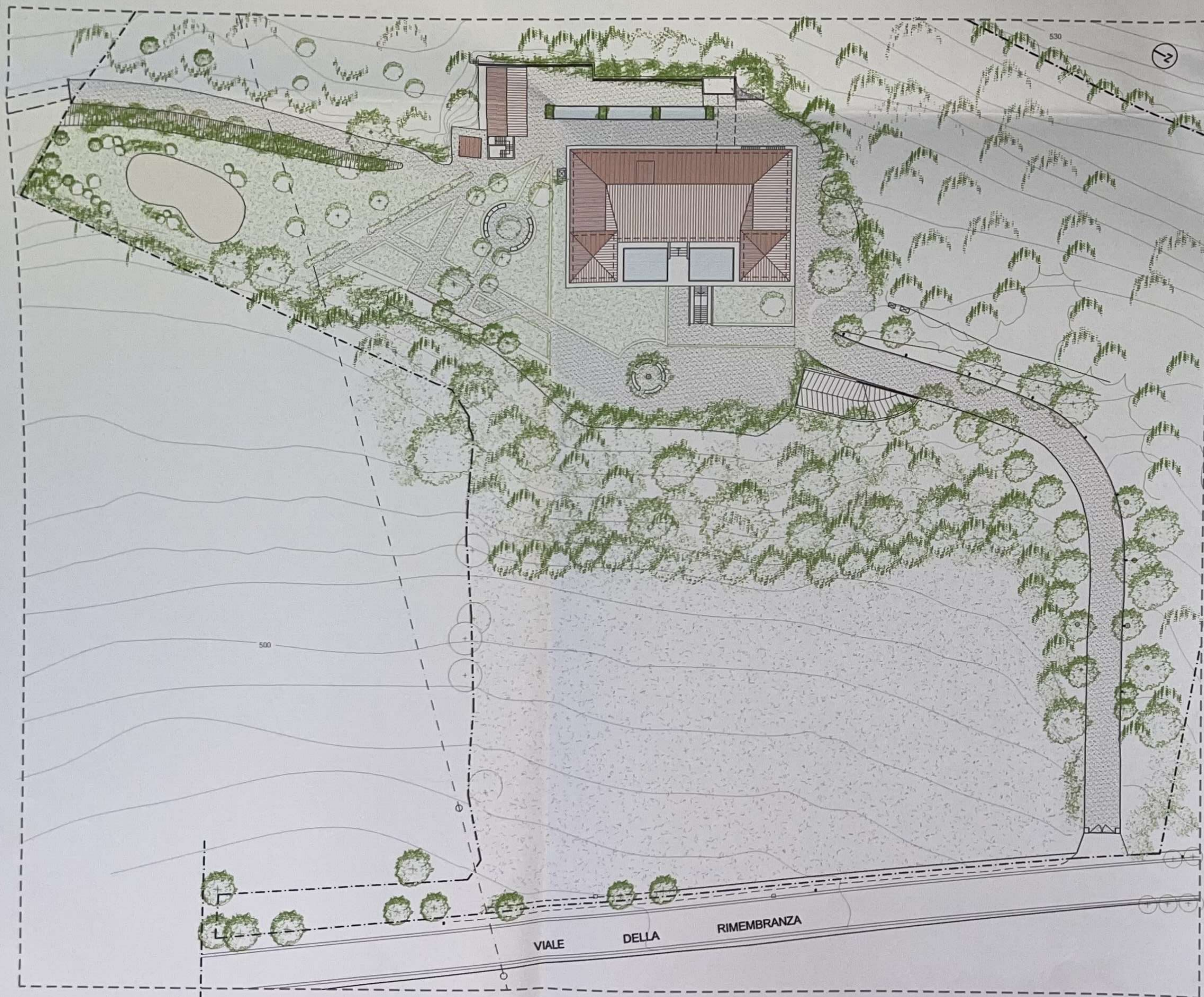
PLANIMETRIA GENERALE SCALA 1:500
