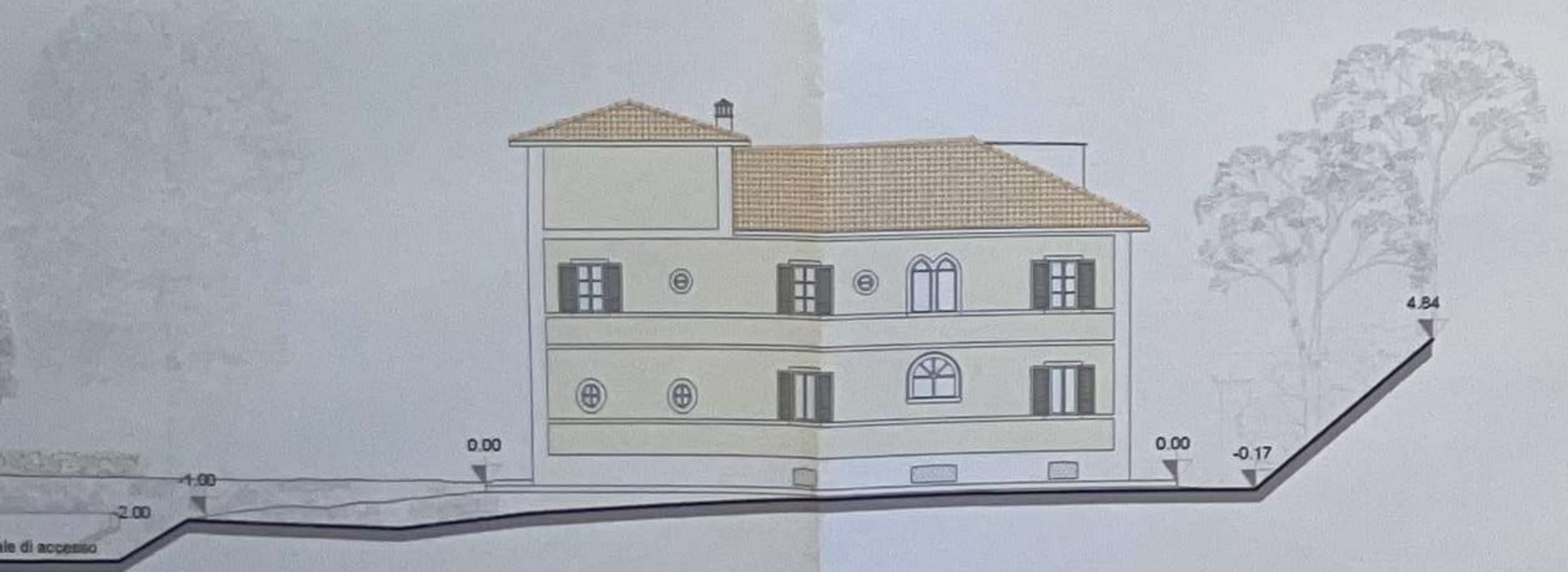
SEZIONE C - C'
